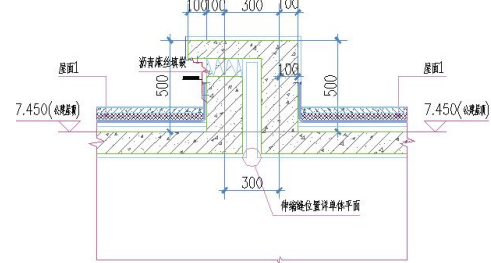
(改良后屋面伸缩缝工艺)
